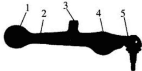
Brazo de soporte (1.4. Casquillo de goma, 2. Cuerpo del brazo de control, 3. Orificio de montaje, 5. Conjunto de rótula)
