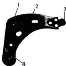
Buje doble, brazo triangular con bisagra de bola simple (1.4. Buje de goma, 2. Cuerpo del brazo, 3. Conjunto de rótula)
