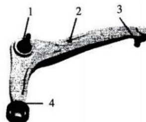
Buje simple, brazo triangular con bisagra de doble bola. (1.3. Conjunto de rótula, 2. Cuerpo del brazo, 4. Casquillo de goma)
